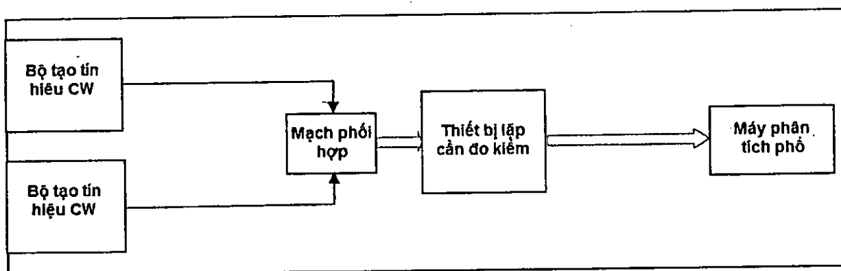
Hình C. 5 – Sơ đồ hệ đo xuyên điều chế đầu vào Chú ý rằng thiết bị lập là thiết bị hai chiều. Bộ tạo tín hiệu có thể cần bảo vệ.
