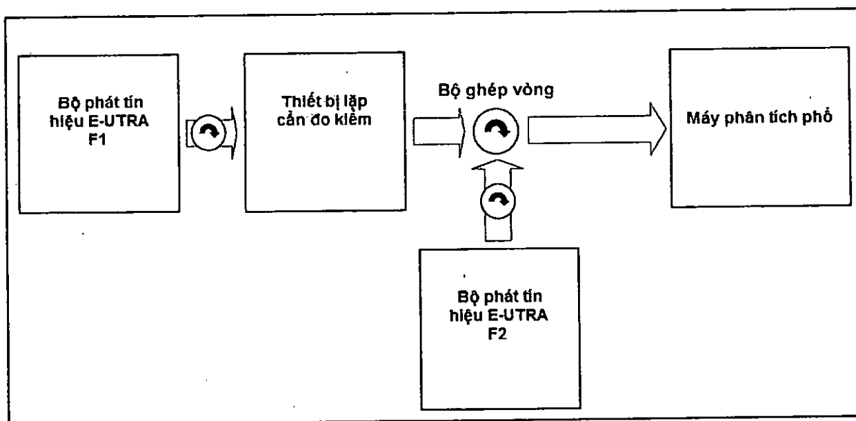
Hình C. 6 – Sơ đồ hệ đo xuyên điều chế đầu ra Chú ý rằng thiết bị lập là thiết bị hai chiều. Bộ tạo tín hiệu có thể cần bảo vệ.
