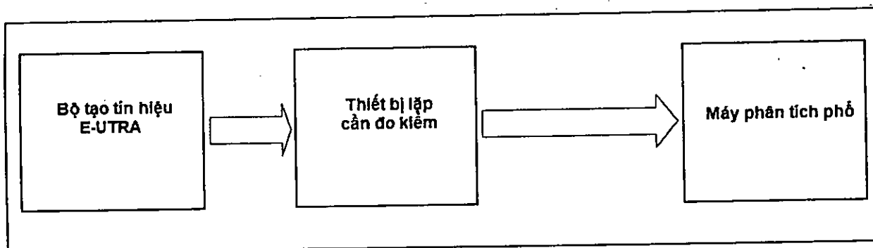
Hình C. 4 – Sơ đồ hệ đo phát xạ không mong muốn: Phát xạ giả Chú ý rằng thiết bị lập là thiết bị hai chiều. Bộ tạo tín hiệu có thể cần bảo vệ.
