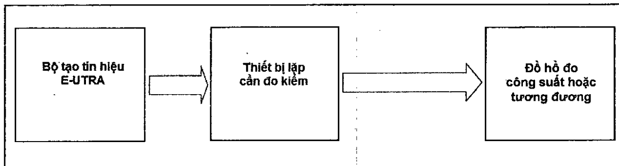
Hình C. 1 – Sơ đồ hệ đo công suất cực đại
